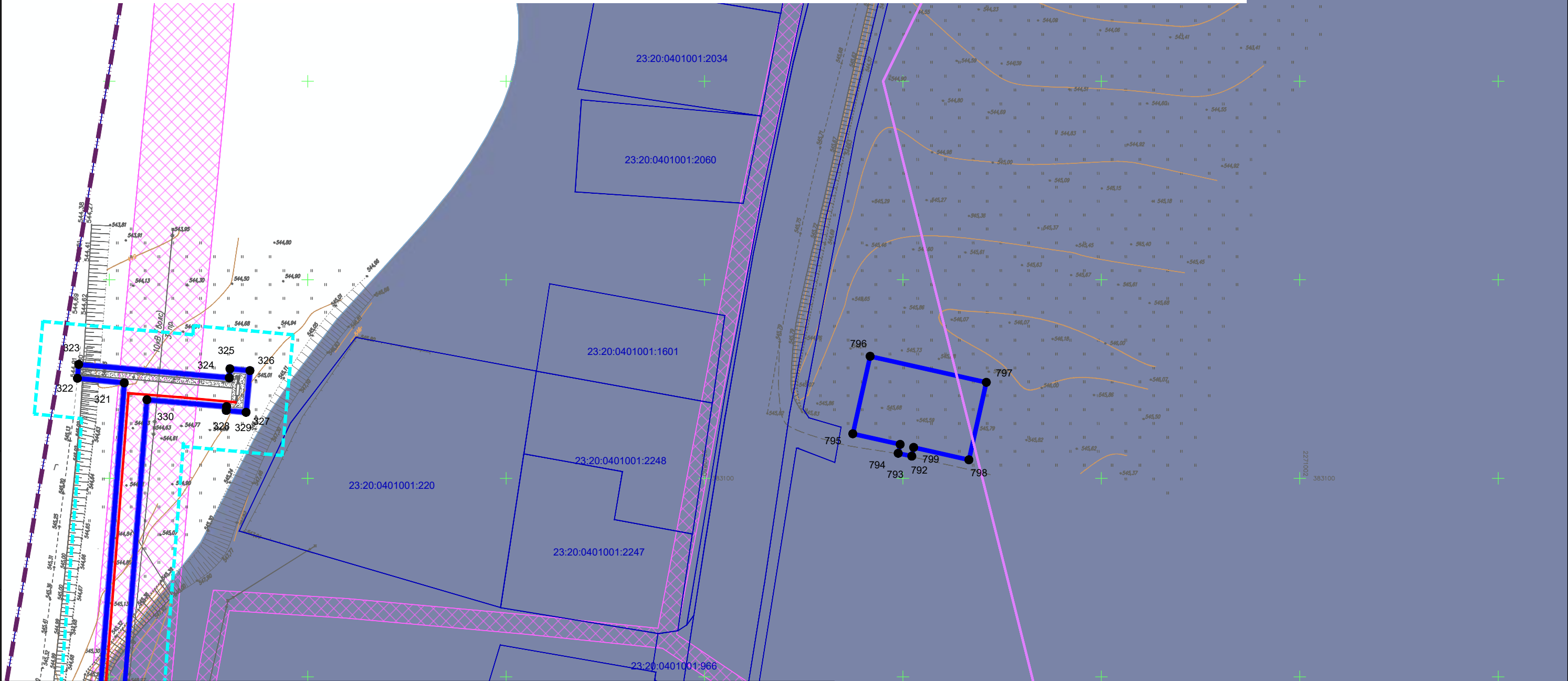
Чертеж межевания территории
